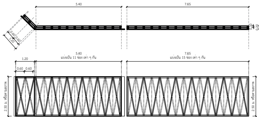
ดูแบบขยายFACADE 2
