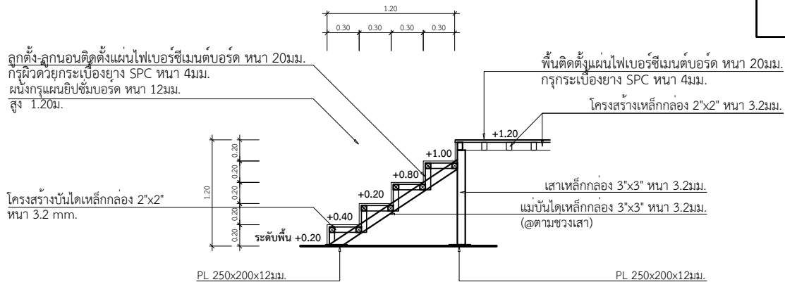
รูปตัดบันไดด้านหลัง มาตราส่วน 1 : 25
