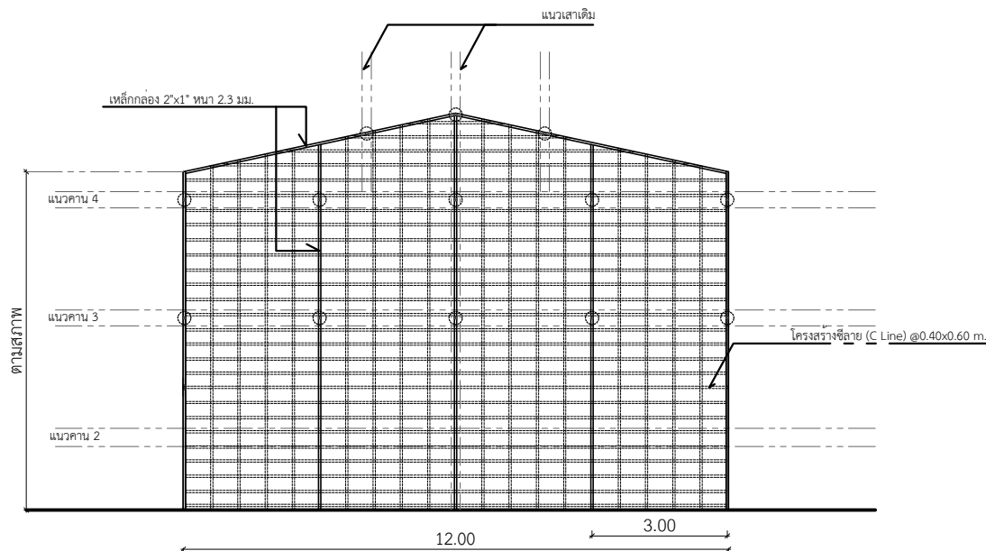
โครงสร้างด้านหน้า มาตราส่วน 1 : 75
