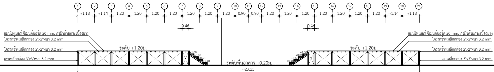
รูปตัด B-01
