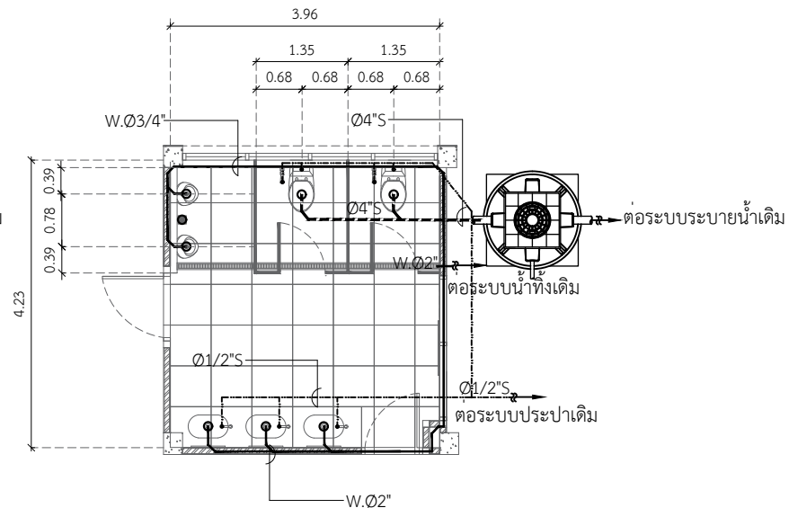
แปลนสุขาภิบาลห้องน้ำชาย
