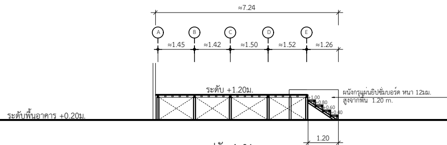
รูปตัด A-01
