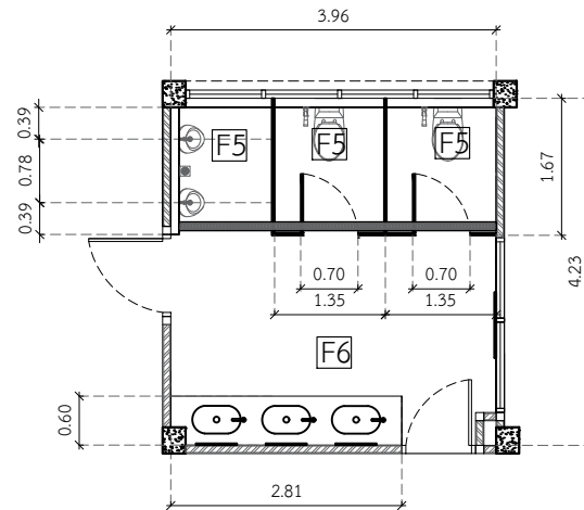
แปลนห้องน้ำชาย
