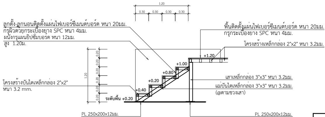
รูปตัดบันไดด้านหน้า มาตราส่วน 1 : 25
