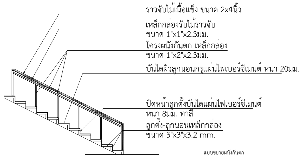
แบบขยายผนังกันตก มาตราส่วน 1 : 50
