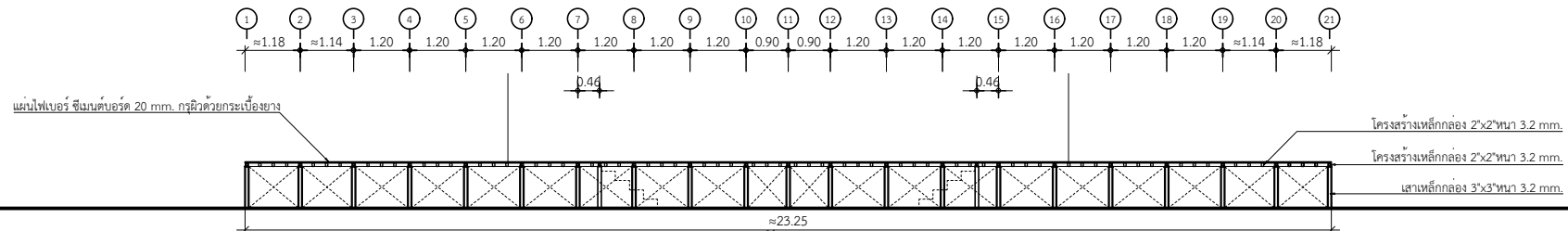
รูปตัด B-02
