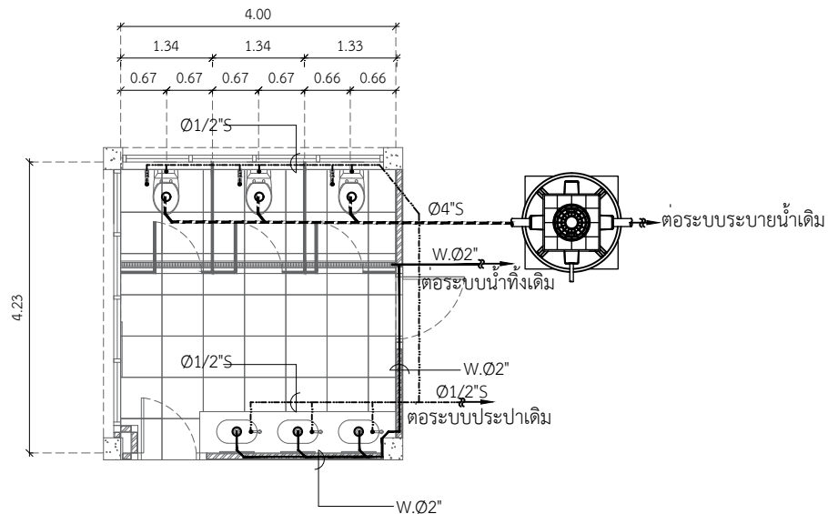
แปลนสุขาภิบาลห้องน้ำใหญ่
