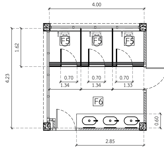
แปลนห้องน้ำหญิง
